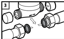
3 Удалите защитные колпачки, установите новые прокладки
