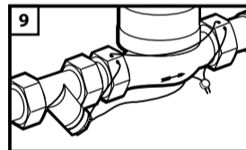
9 Опломбируйте счетчик и фильтр в установленных местах
